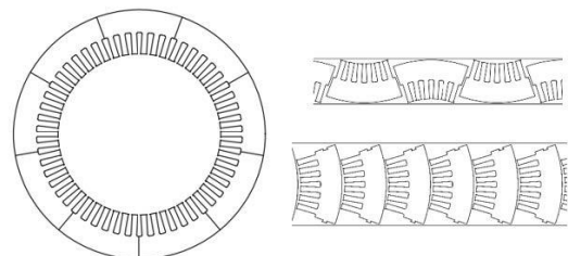
Bild 1: Stator und Statorsegmente Beispiel
